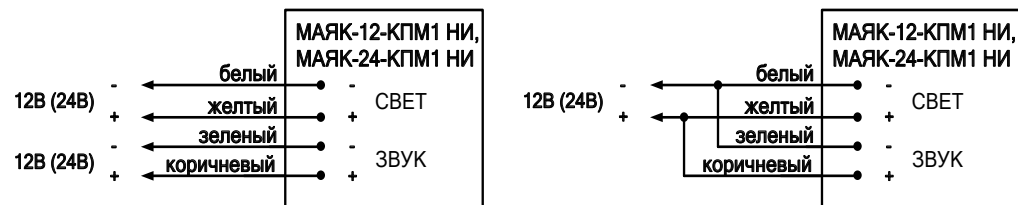
Рис.1. Схема подключения.
