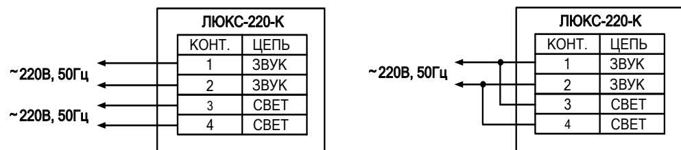
Рис.1. Схемы подключения.
