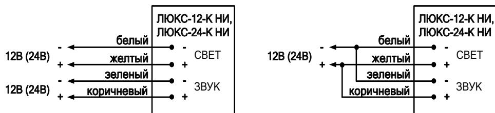
Рис.1. Схема подключения.
