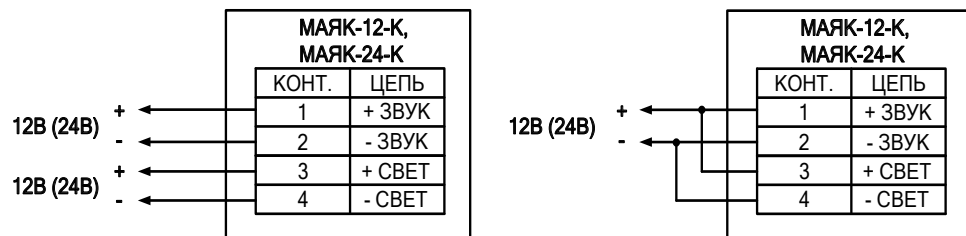
Рис.1. Схема подключения.
