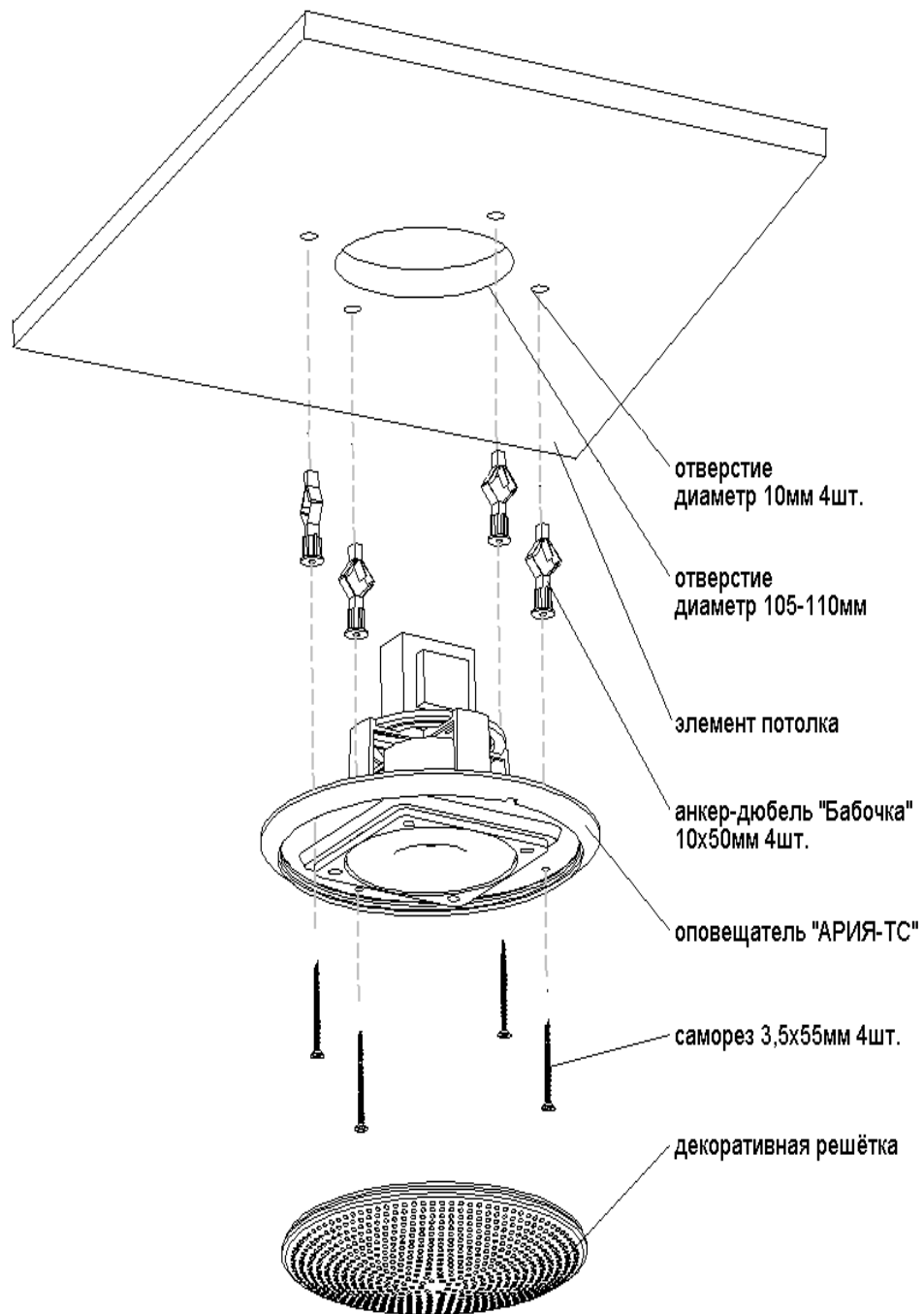
Рис.2. Монтажная схема.
