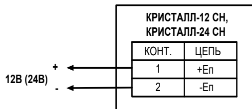
Рис.1. Схема подключения.
