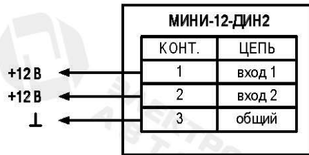
Рис.1. Схема подключения.
