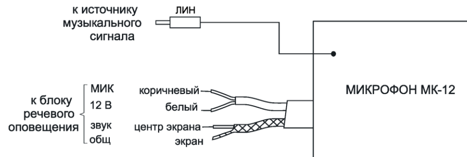
Рис.1. Схема соединений микрофона при подключении с максимальным приоритетом.
