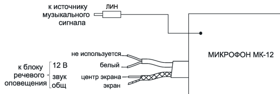
Рис.2. Схема соединений микрофона при подключении с минимальным приоритетом.
