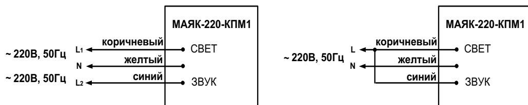
Рис.1. Схема подключения.
