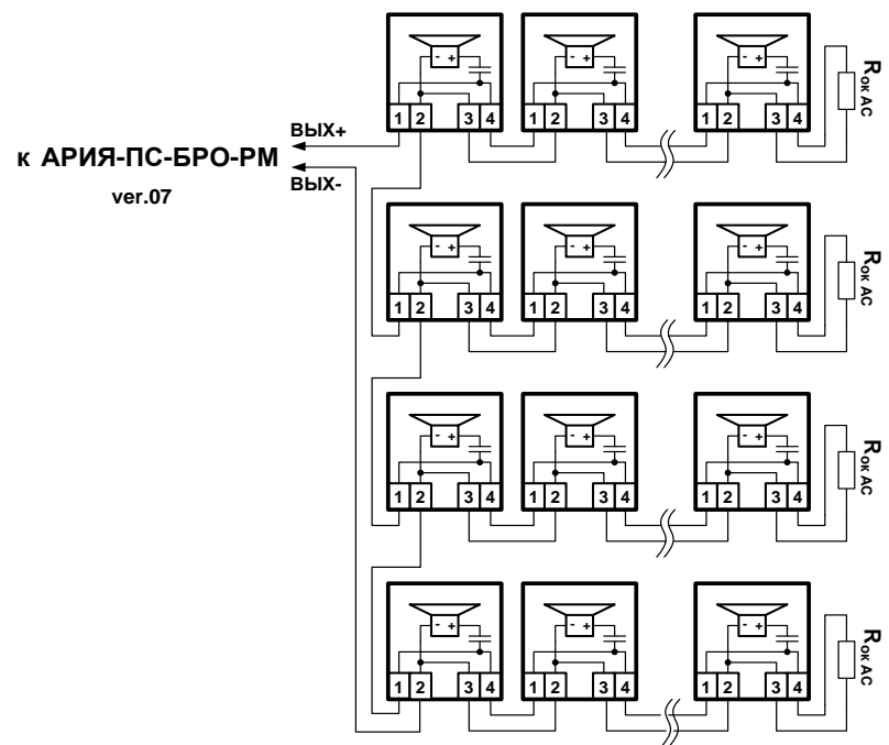
Г. Схема соединений 8, 12, 16, 20, 24, 28, 32, 36, 40, 44 и 48 речевых оповещателей серии АРИЯ-ПС. Номинал оконечного резистора R ок AC =2,4 кОм ± 5%.
