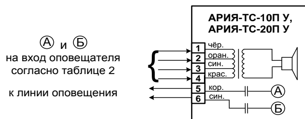
Рис. Схема подключения
