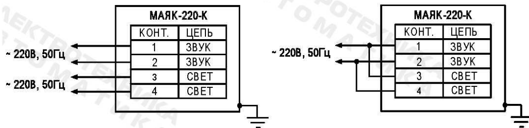
Рис.1. Схема подключения.
